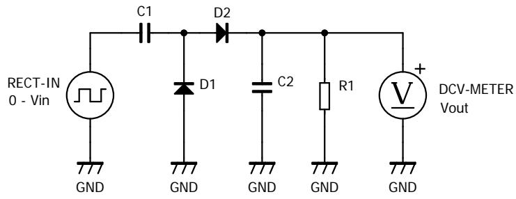
檢波整流回路
